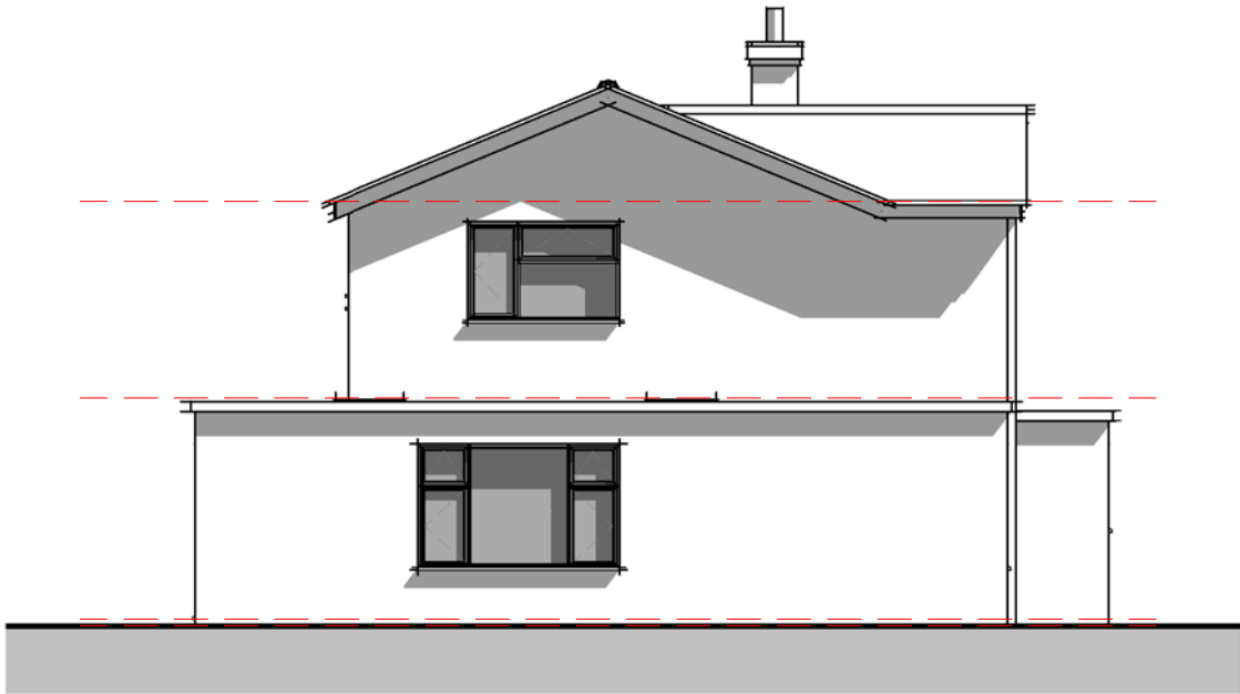
04 - Left Flank 1 : 100
