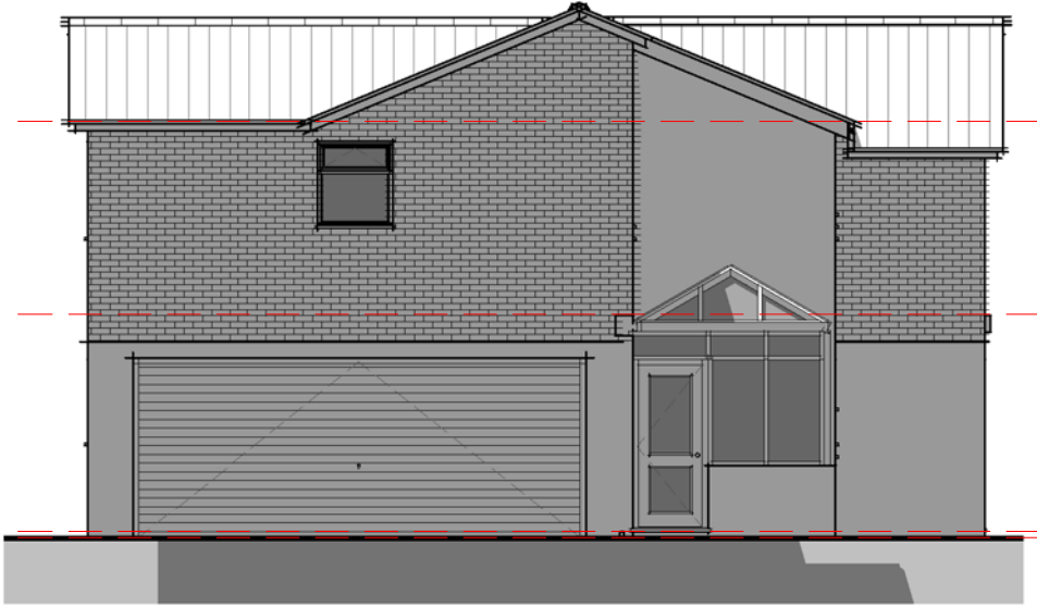
02 - Right Flank 1 : 100
