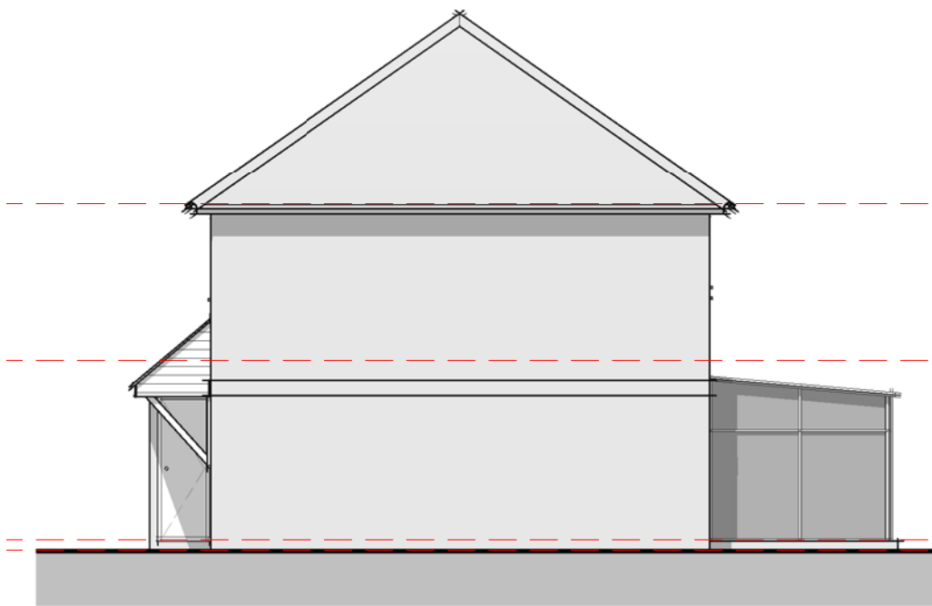
02 - Right Elevation
