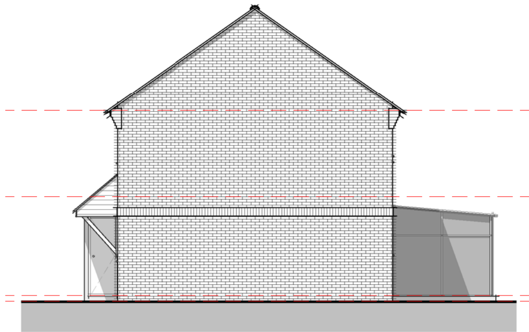
02 - Right Elevation
