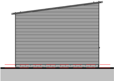
Elevation 04 - Left 1 : 100
