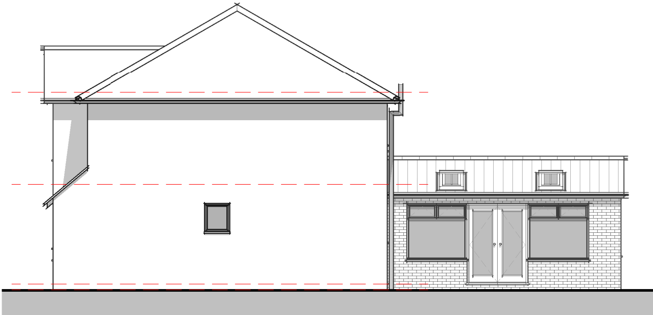
Elevation 02 - Right 1 : 100
