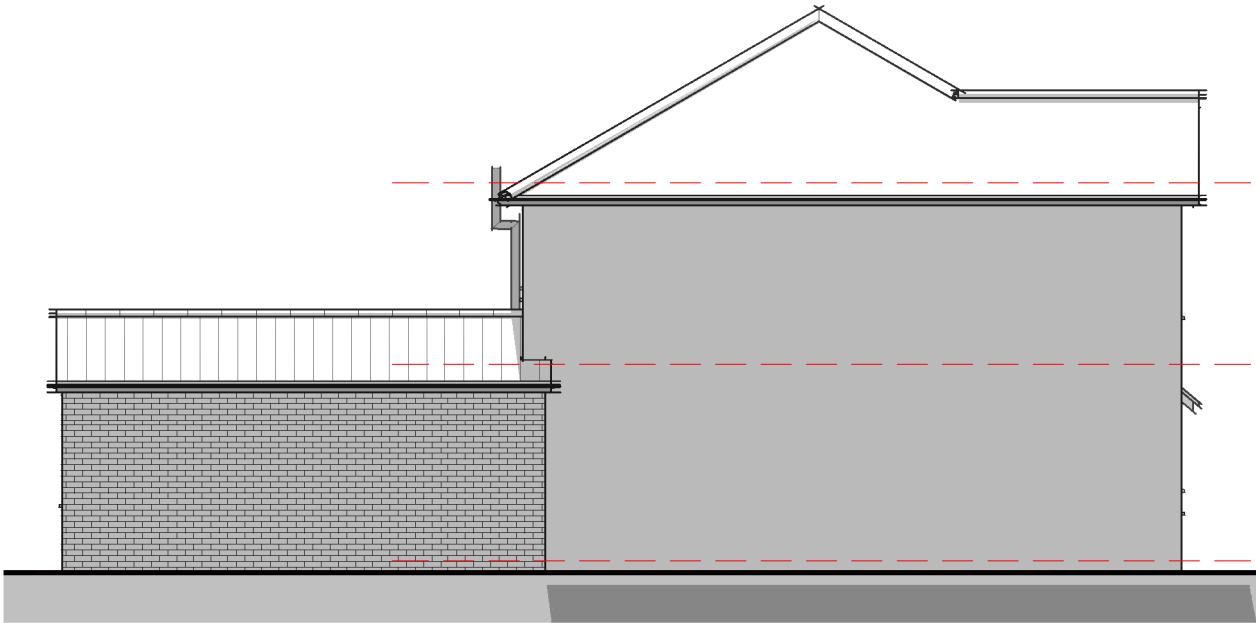
Elevation 04 - Left 1 : 100
