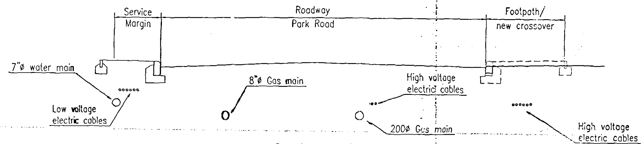
Section A-A
