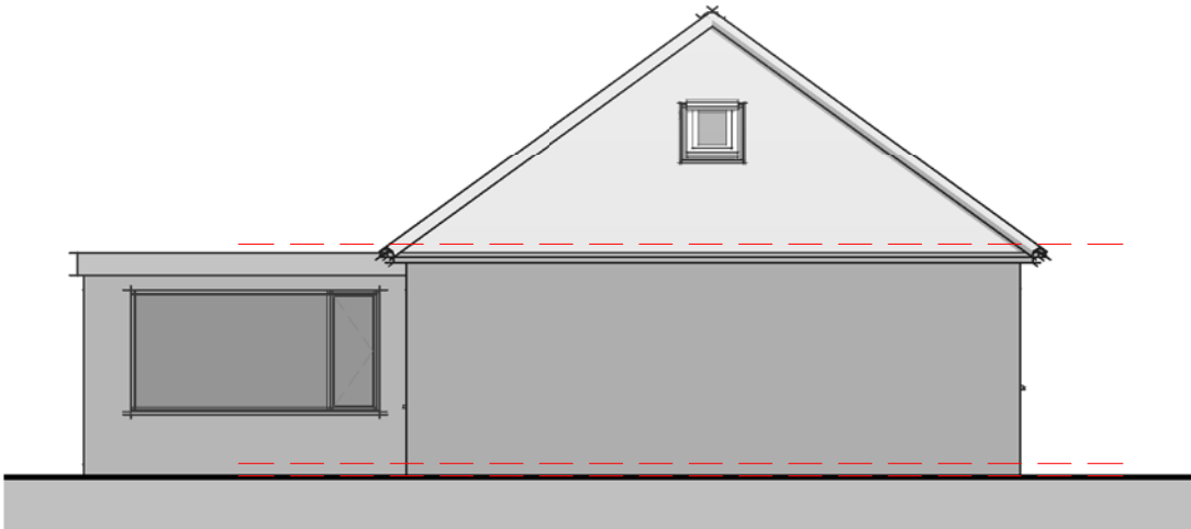
Elevation 04 - Left 1 : 100
