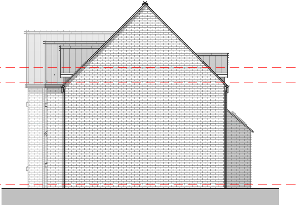
Elevation 02 - Right 1 : 100
