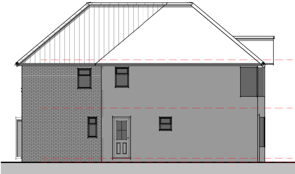
04 - Left Flank 1 : 100
