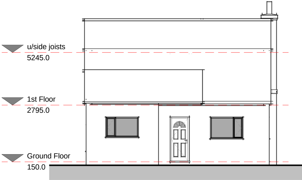
01 - Front 1 : 100
