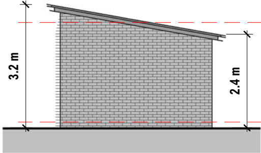
Elevation 02 - Right I : 100
