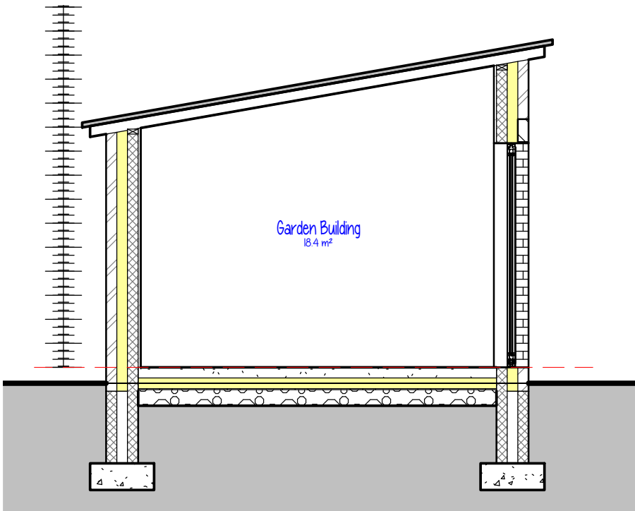
Section I I : 50
