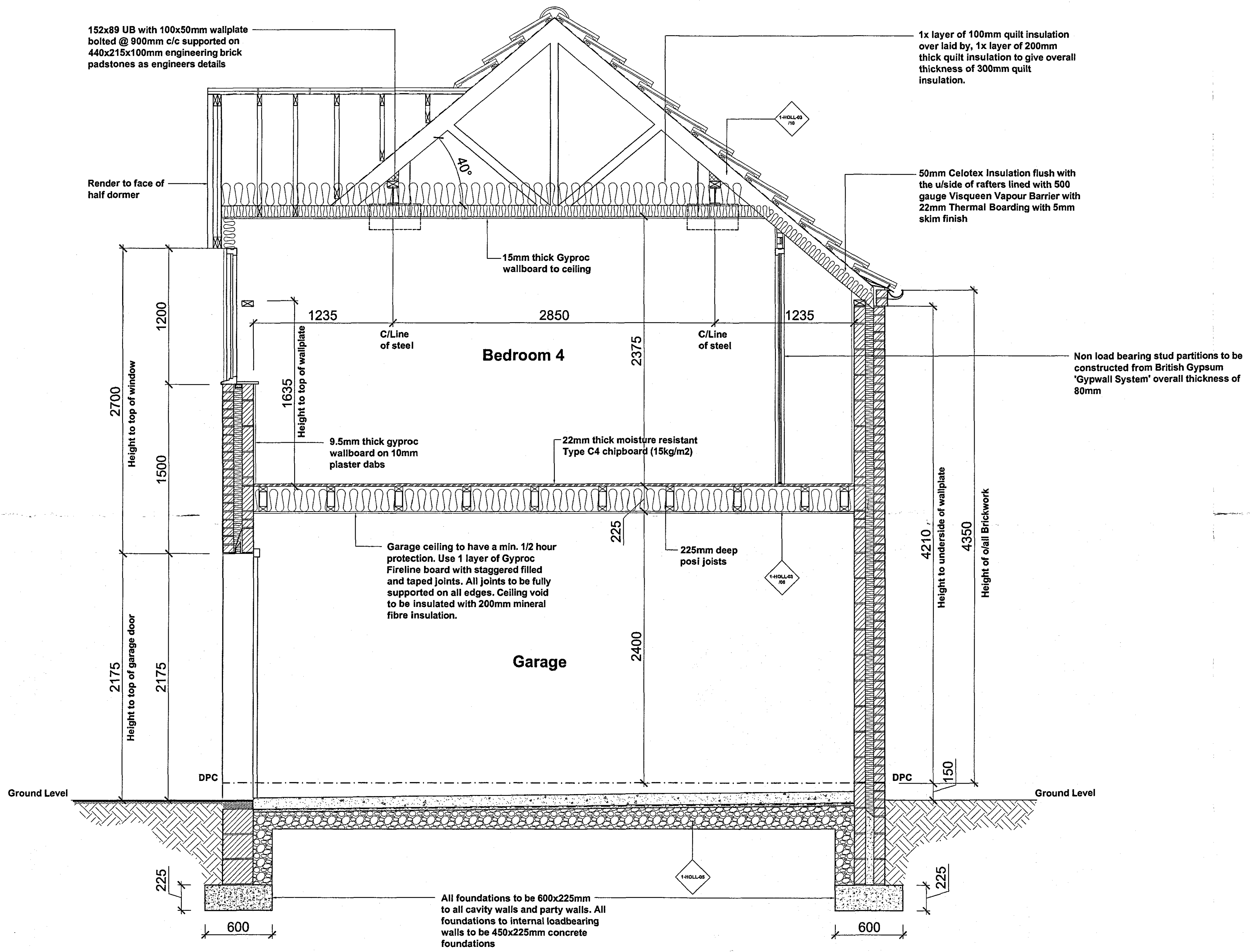
Section A-A
