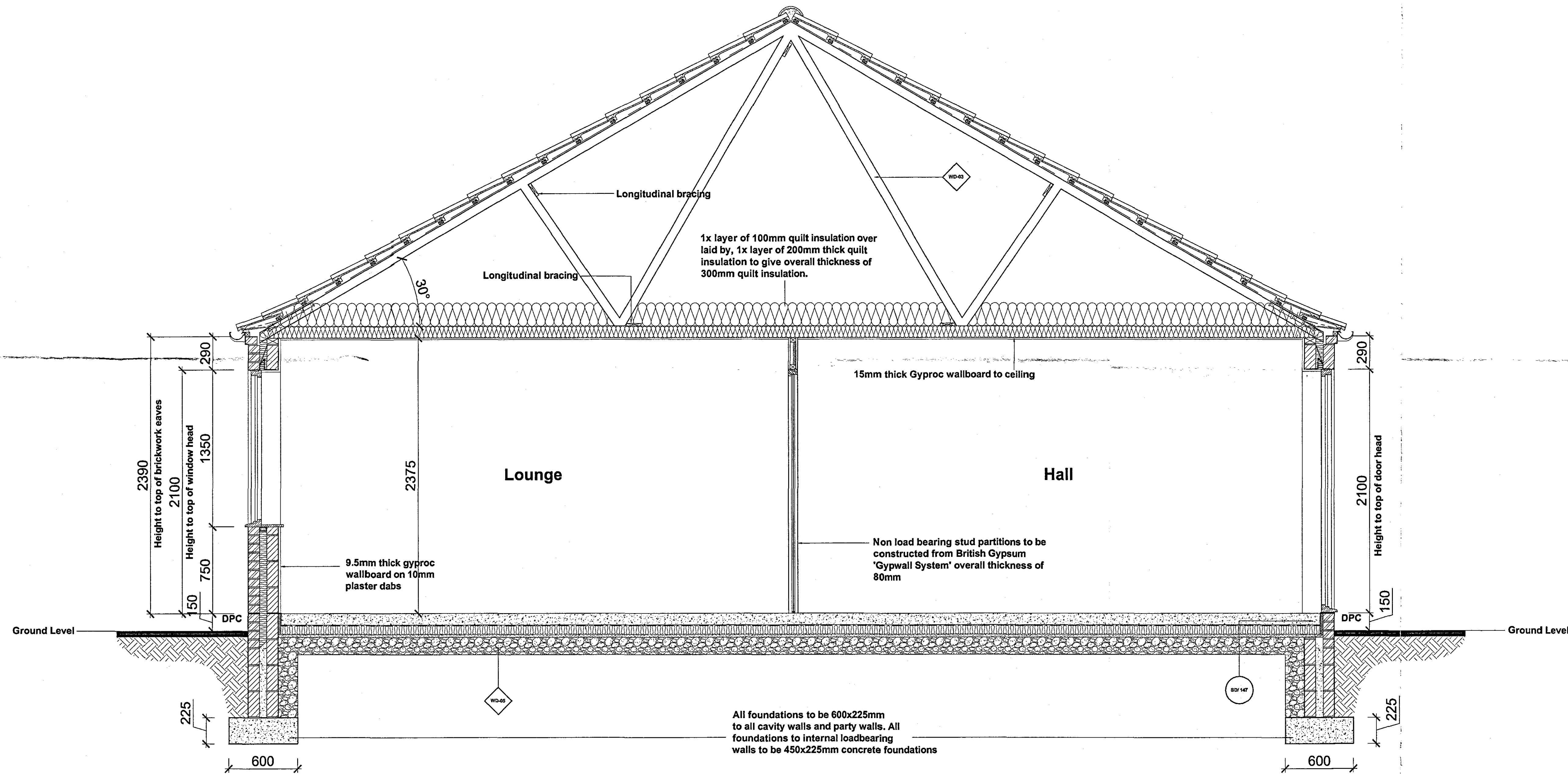
Section A-A
