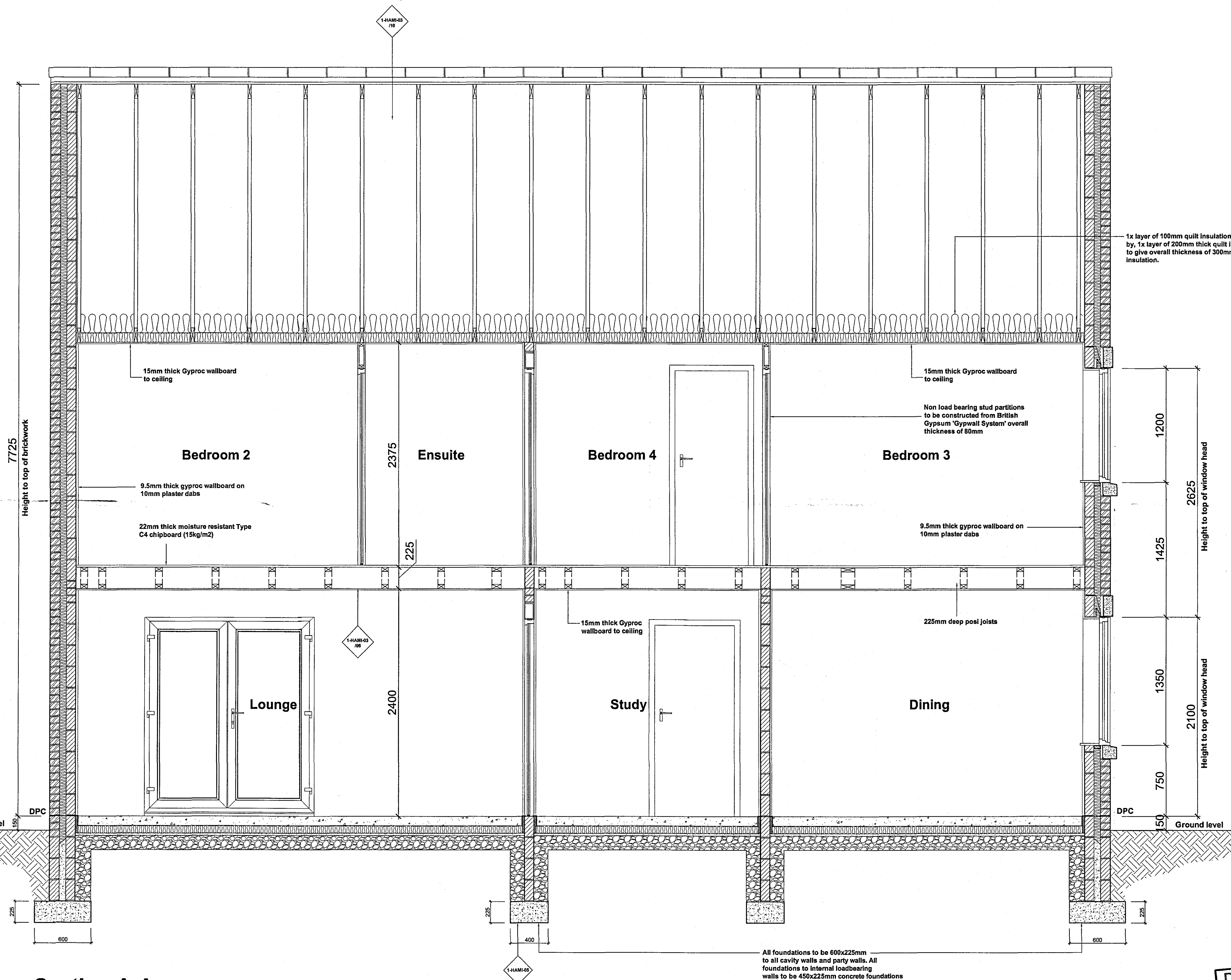
Section A-A
