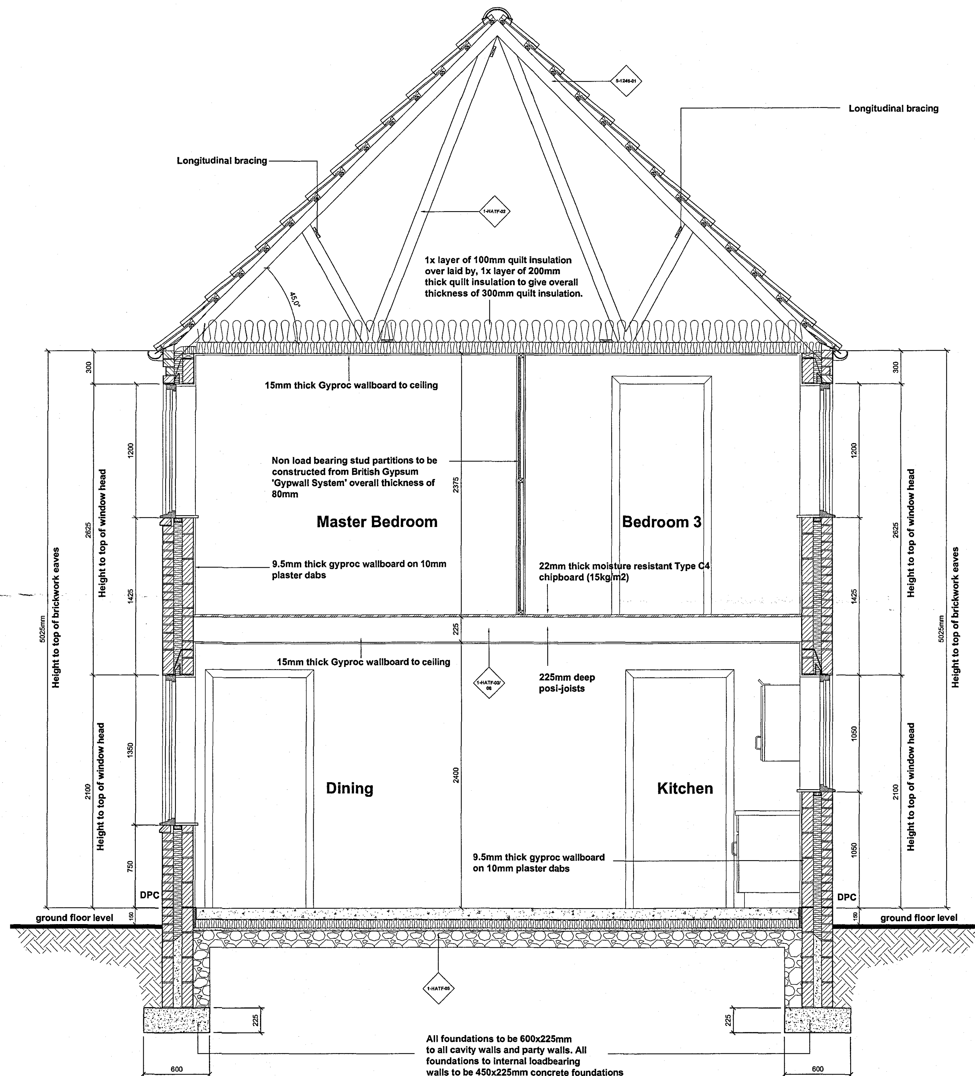
Section A-A
