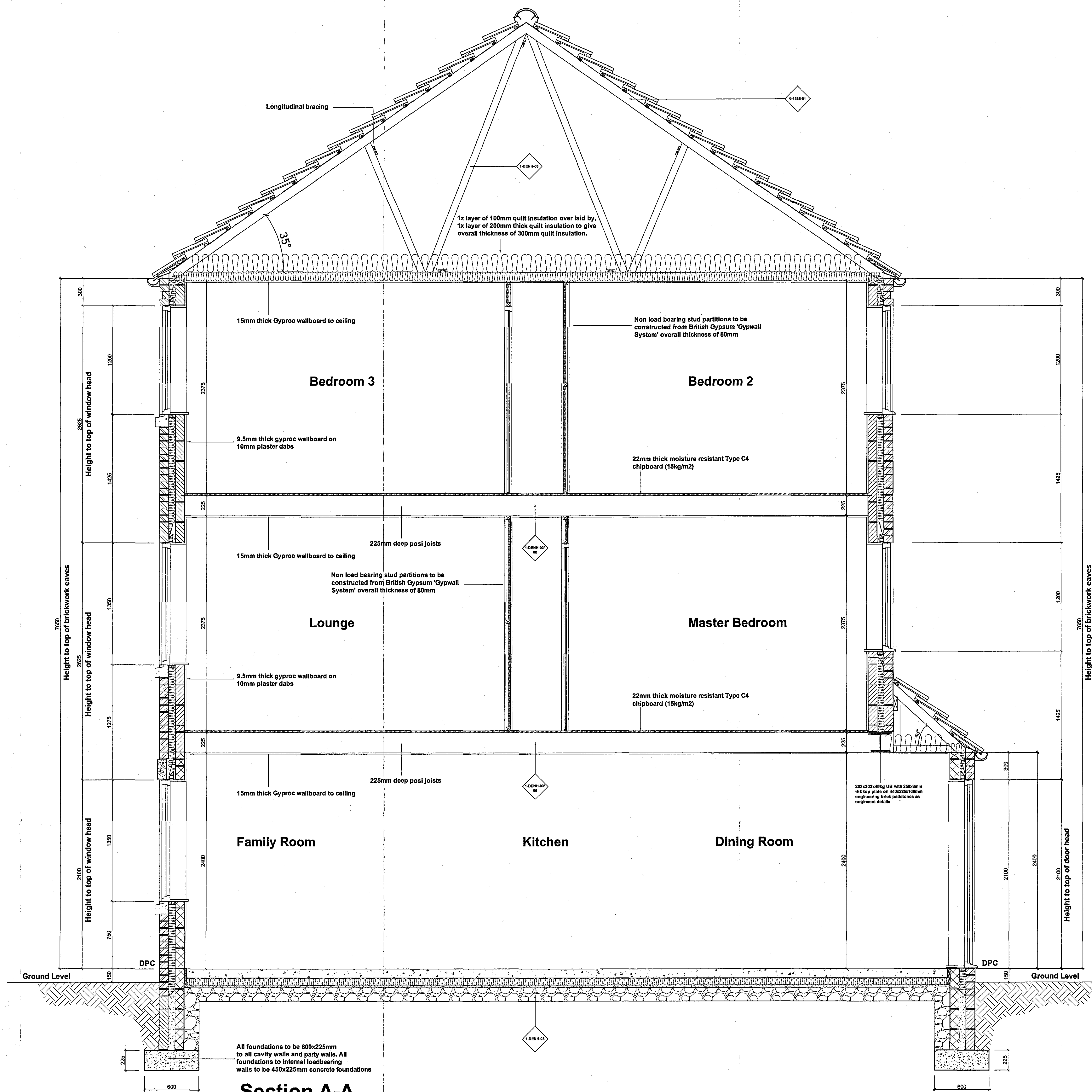
Section A-A
