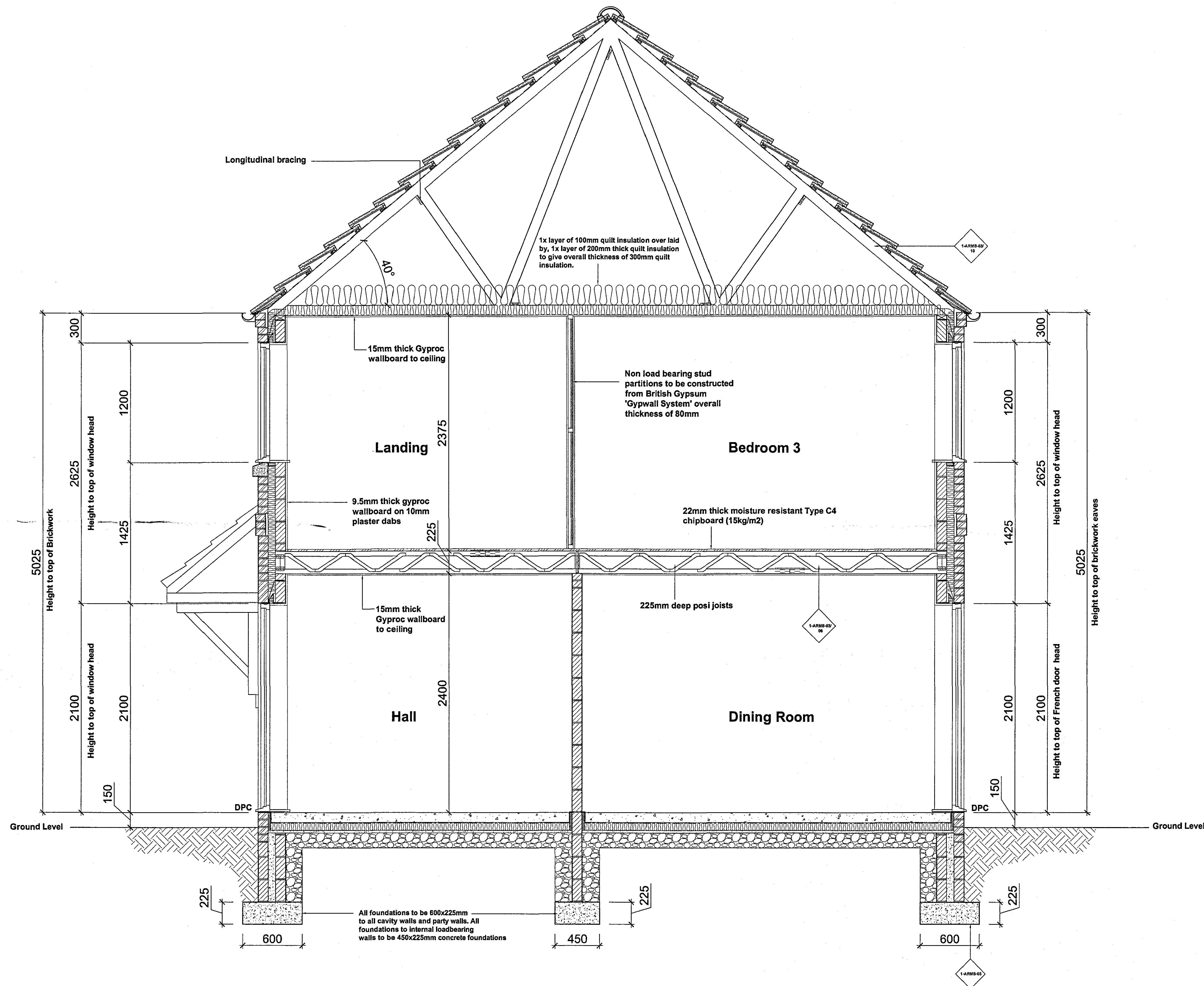
Section A-A
