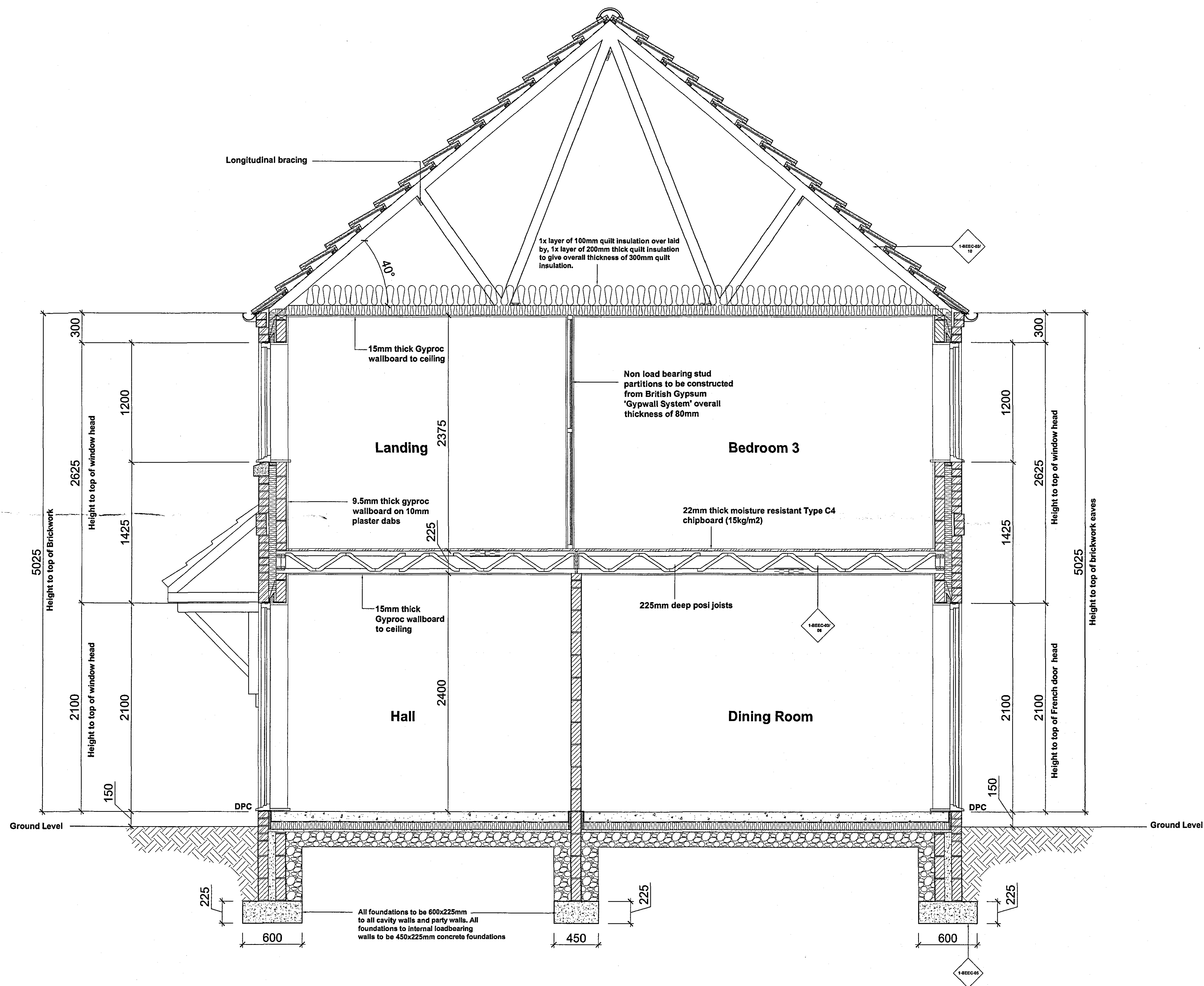
Section A-A
