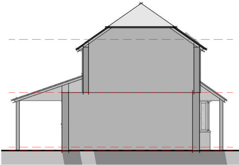
Elevation 04 - Left 1 : 100
