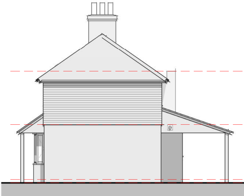
Elevation 02 - Right 1 : 100
