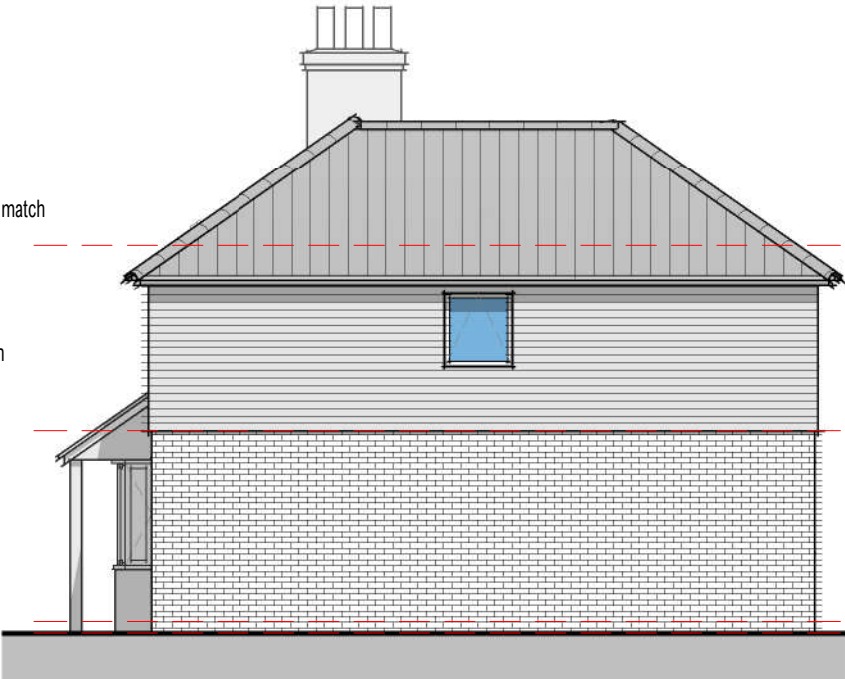
Elevation 02 - Right 1 : 100
