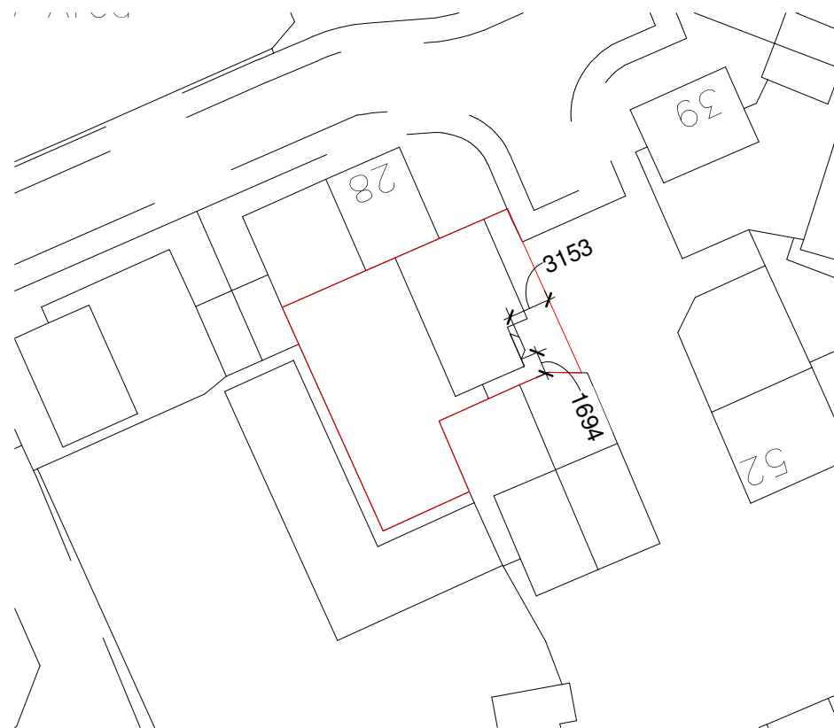
Block Plan 1 : 500
