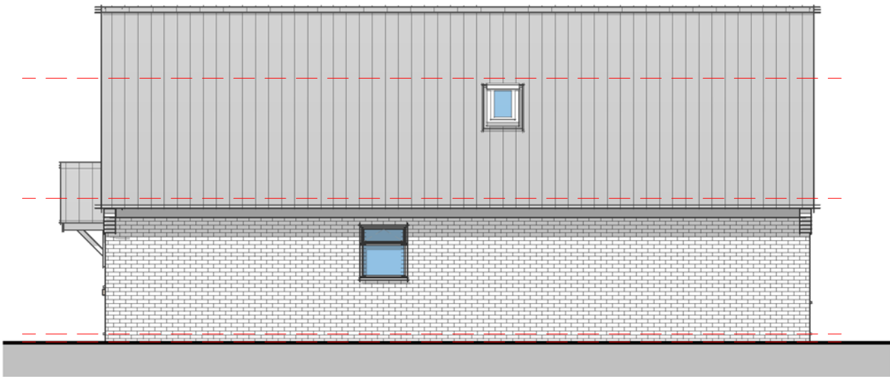
Elevation 02 - Right 1 : 100
