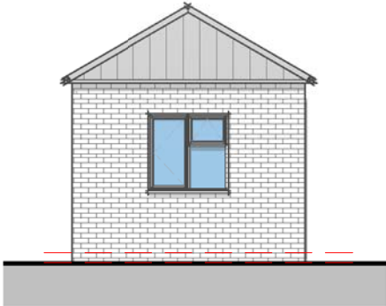
Elevation 02 - Right 1 : 100
