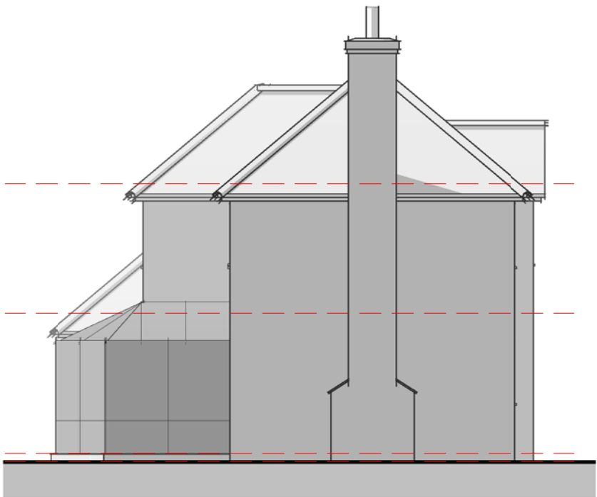
Elevation 04 - Left 1 : 100
