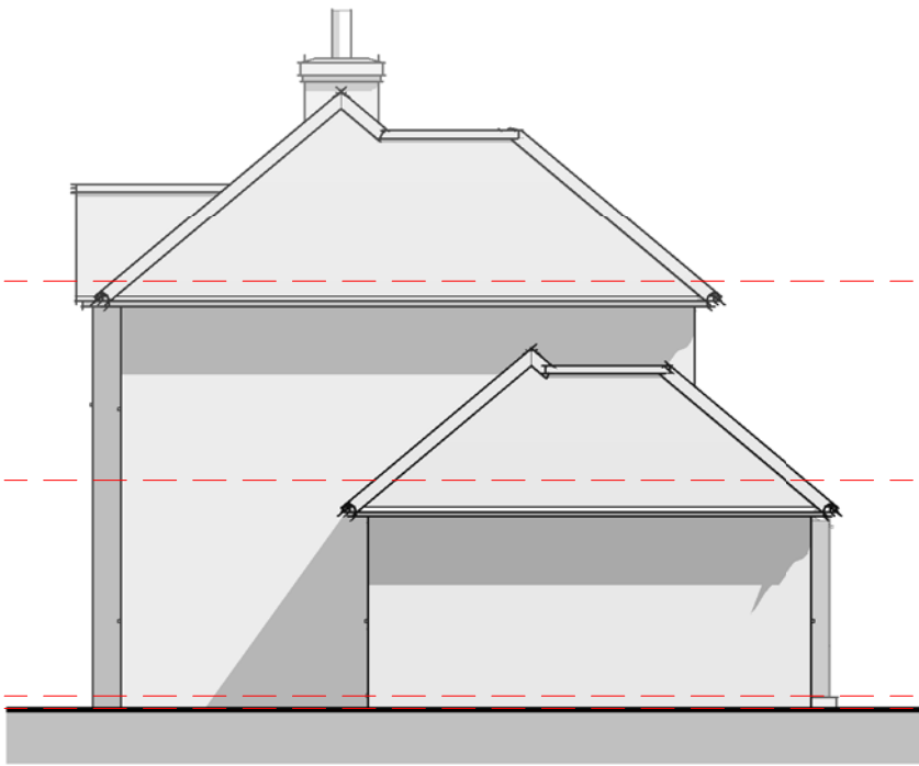
Elevation 02 - Right 1 : 100
