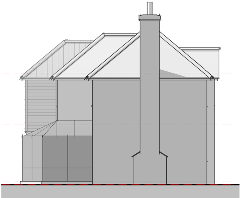
Elevation 04 - Left 1 : 100
