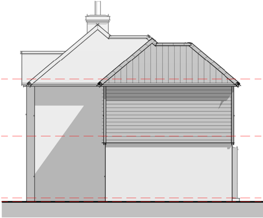
Elevation 02 - Right 1 : 100
