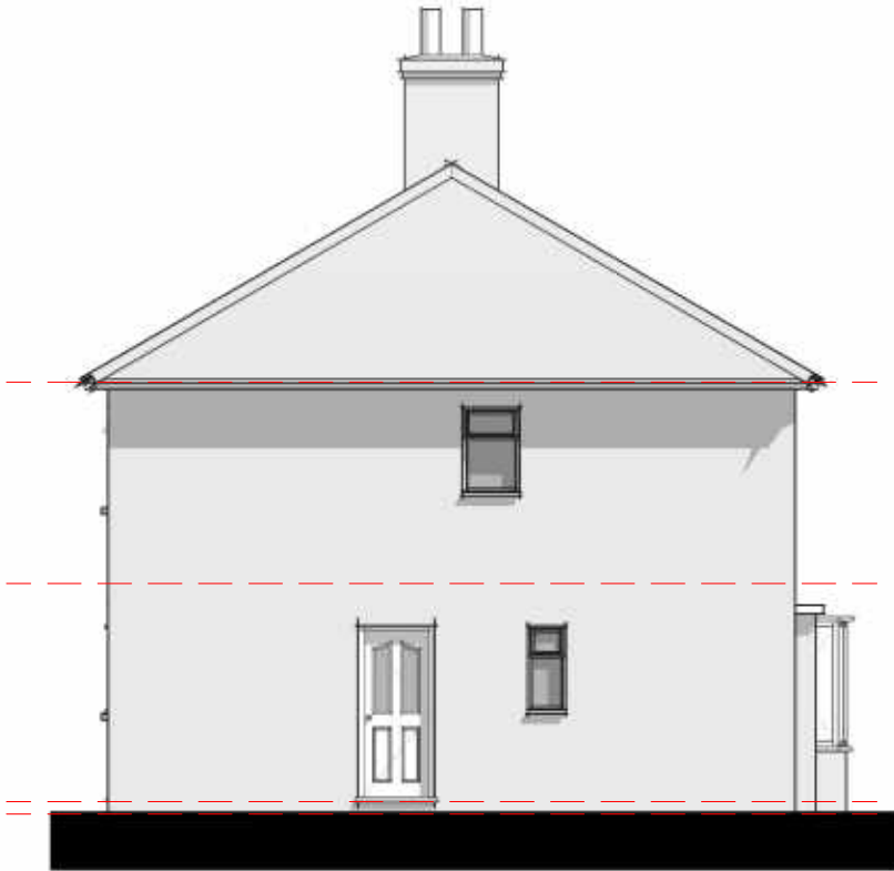
Elevation 04 - Left 1 : 100
