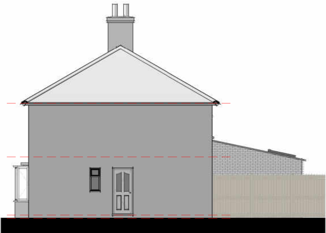
Elevation 02 - Right 1 : 100
