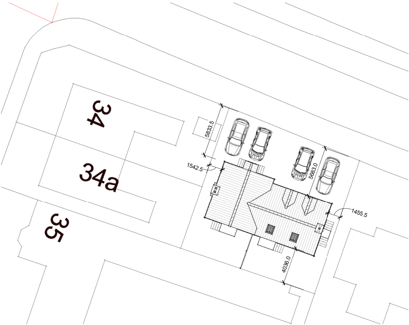
Site Block Plan 1 : 250
