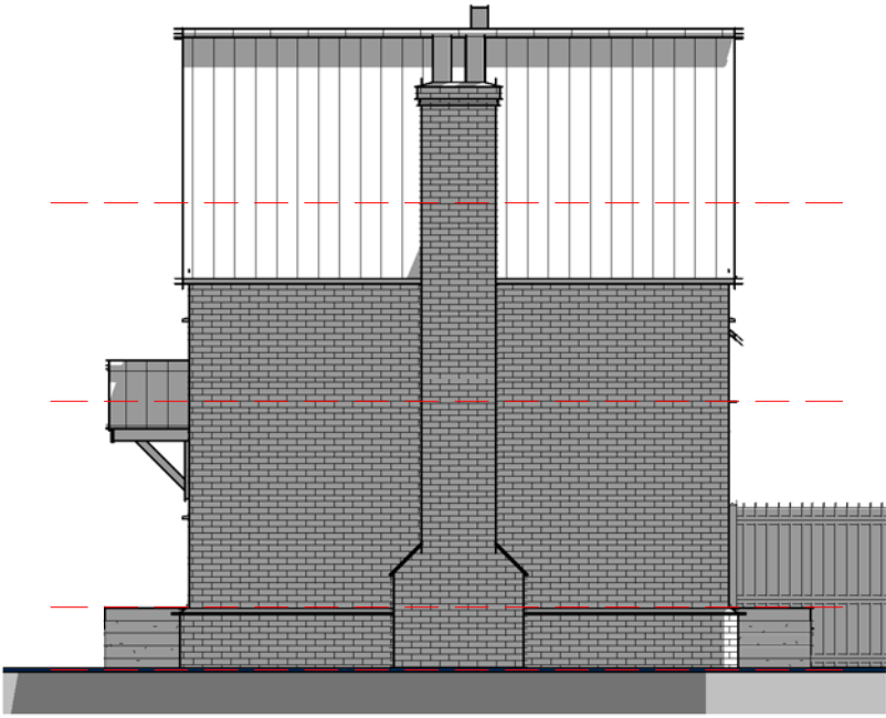
02 - Right Flank 1 : 100
