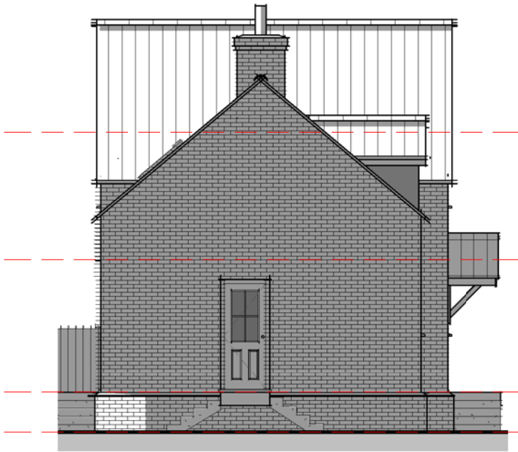
04 - Left Flank 1 : 100
