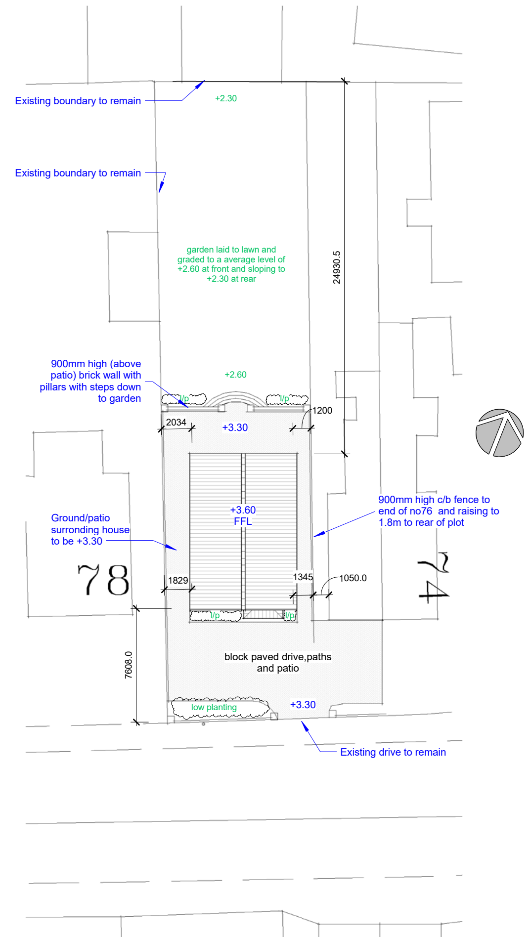
Site Block Plan 1 : 250
