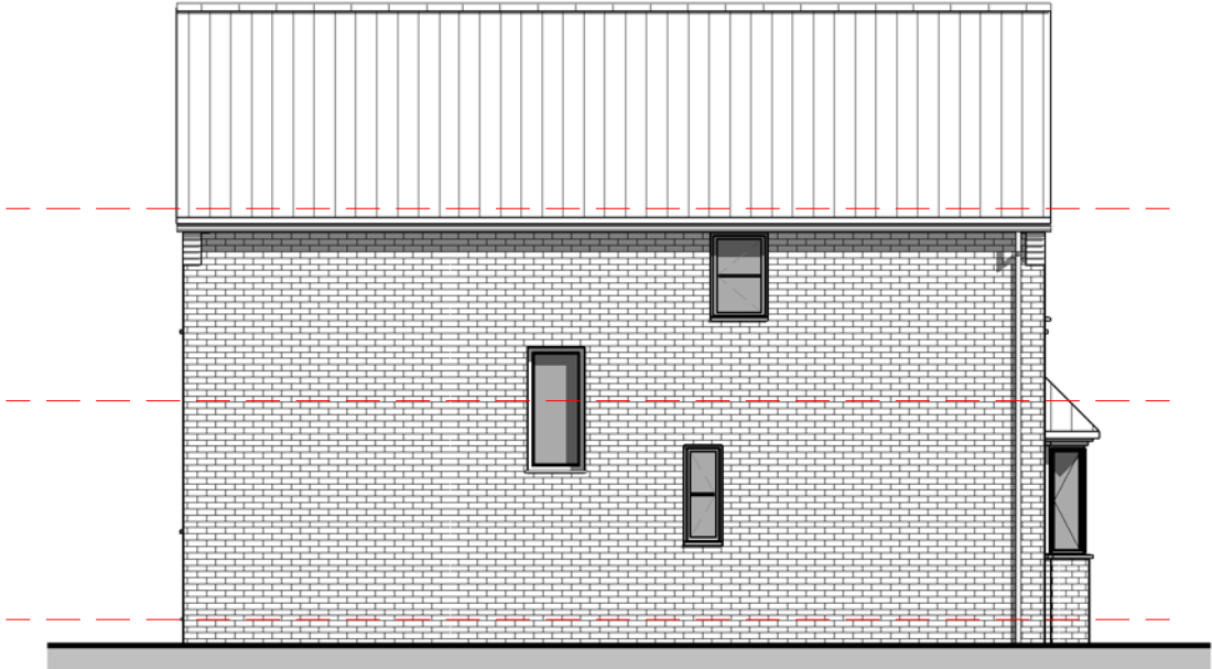
04 - Left Flank 1 : 100
