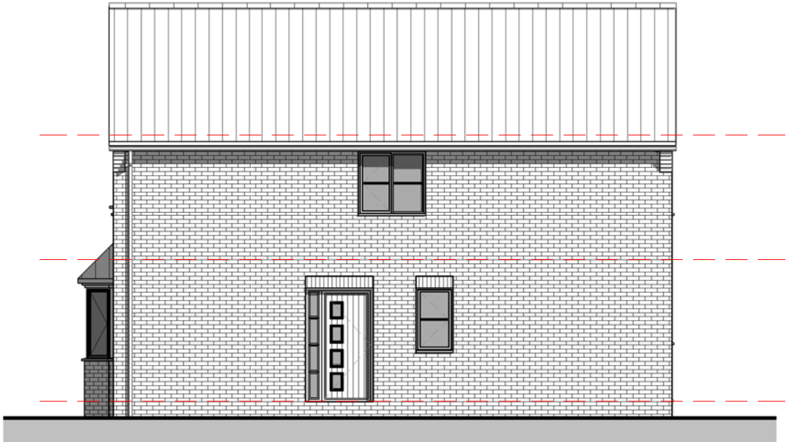
02 - Right Flank 1 : 100
