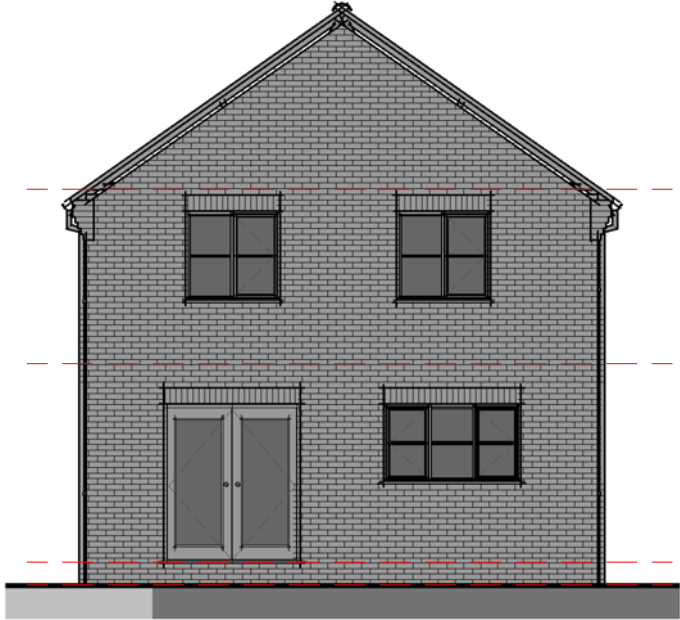
03 - Rear 1 : 100
