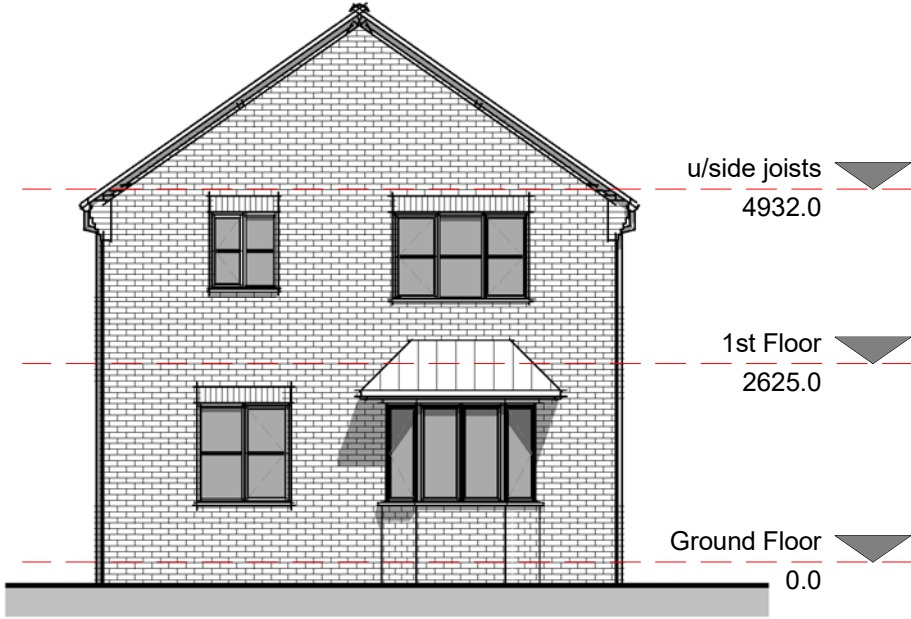
01 - Front 1 : 100
