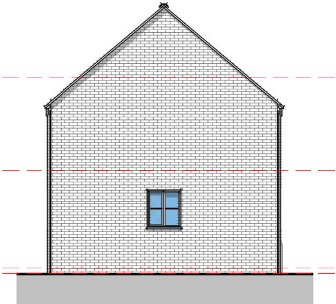
04 - Left Flank 1 : 100
