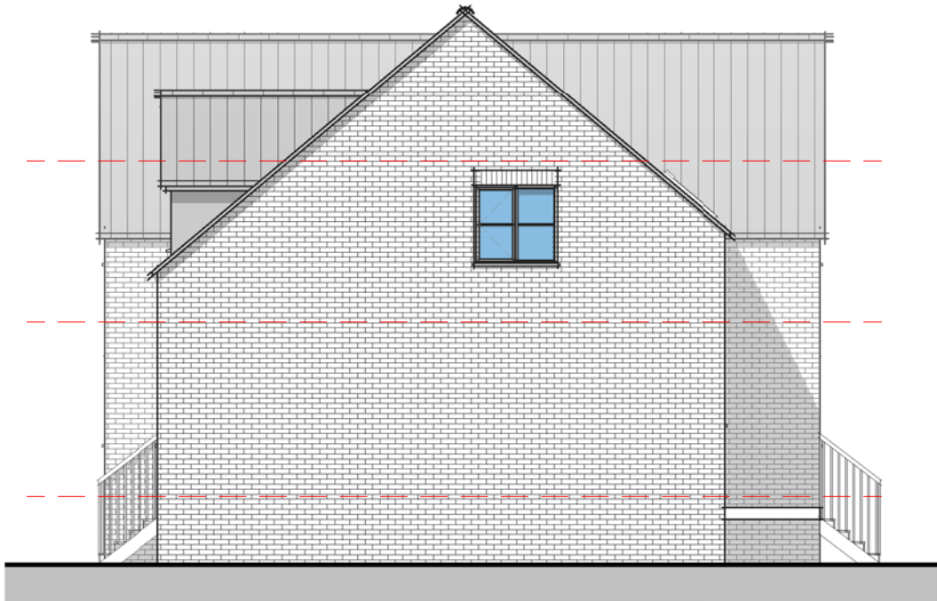
Elevation 02 - Right 1 : 100
