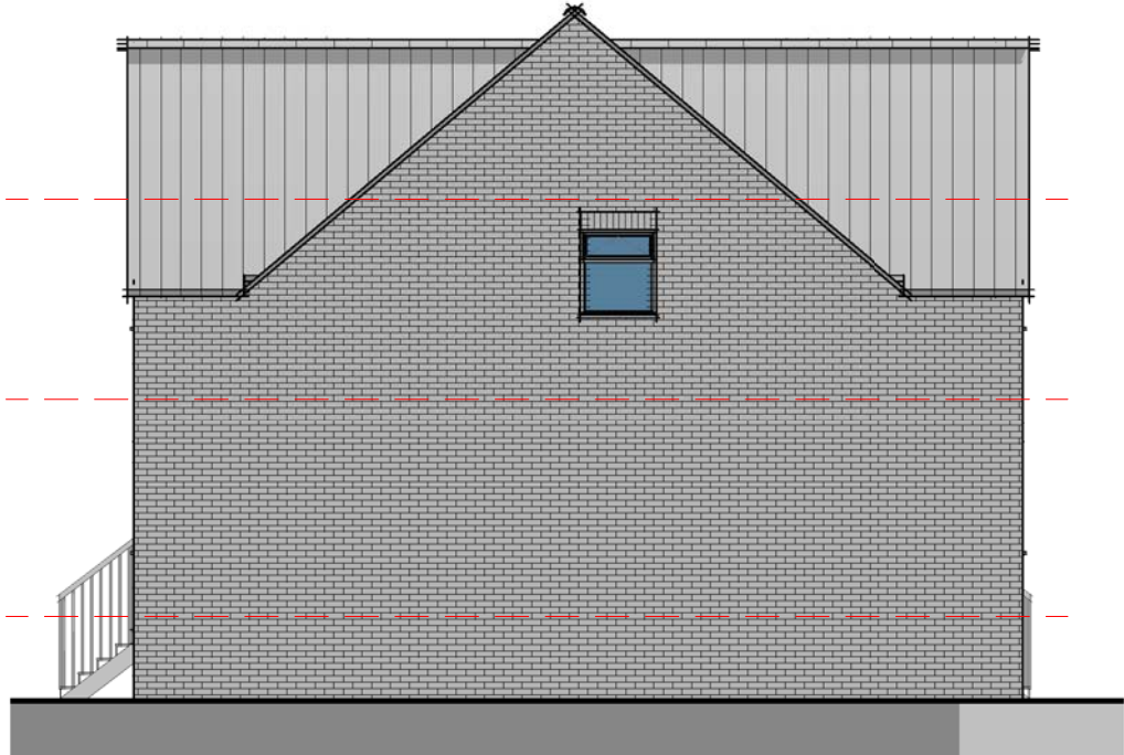
Elevation 04 - Left 1 : 100
