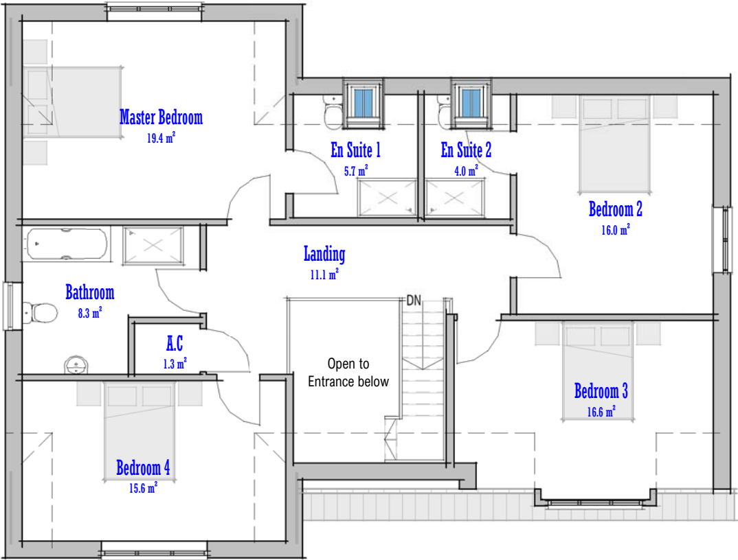
Plan 02 - First 1 : 100
