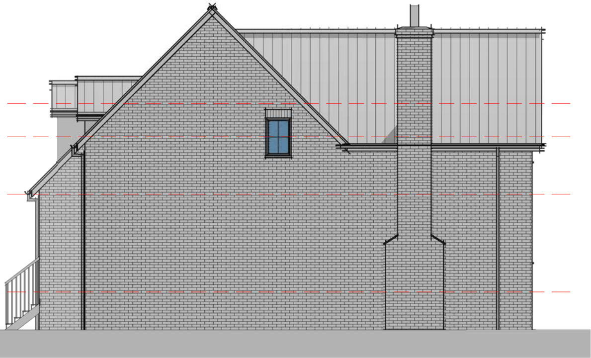
Elevation 04 - Left 1 : 100
