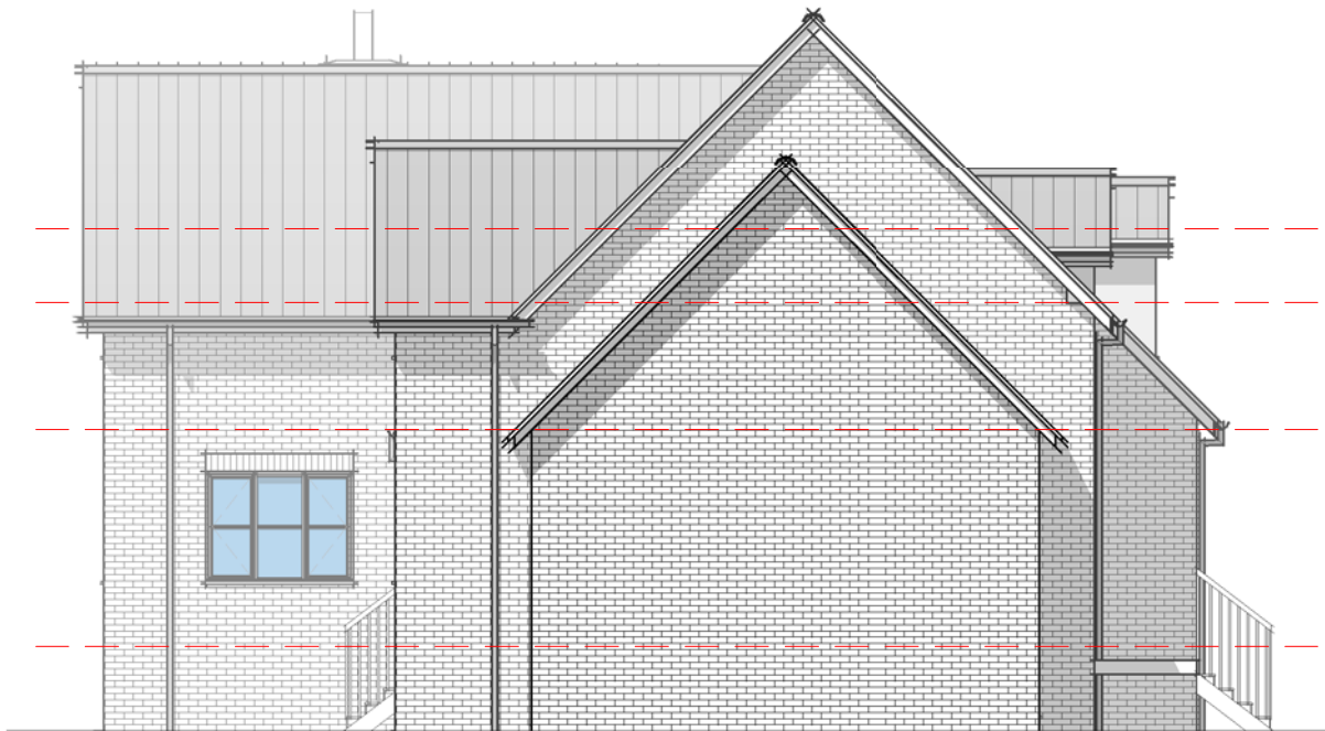
Elevation 02 - Right 1 : 100
