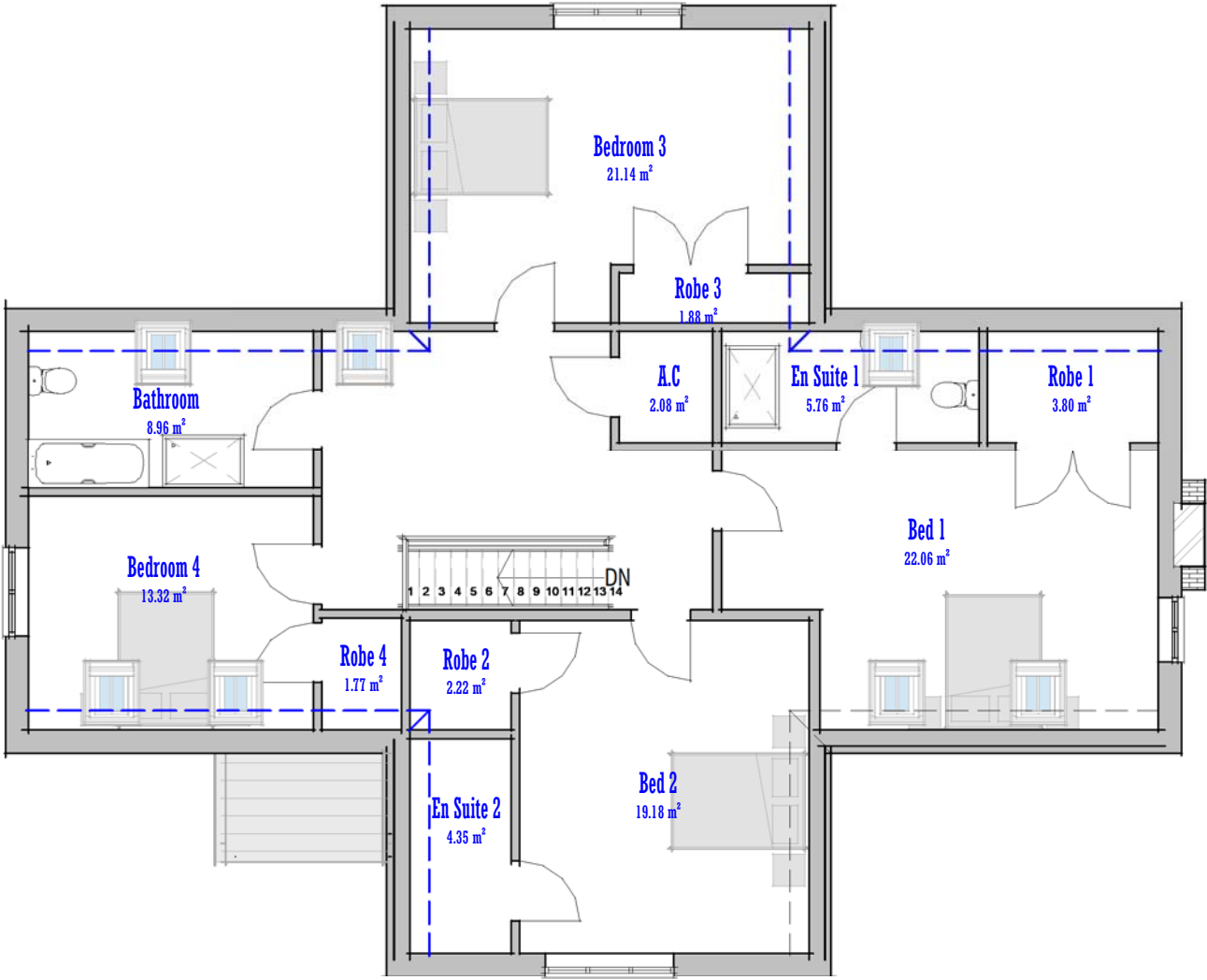
Plan 02 - First 1 : 100
