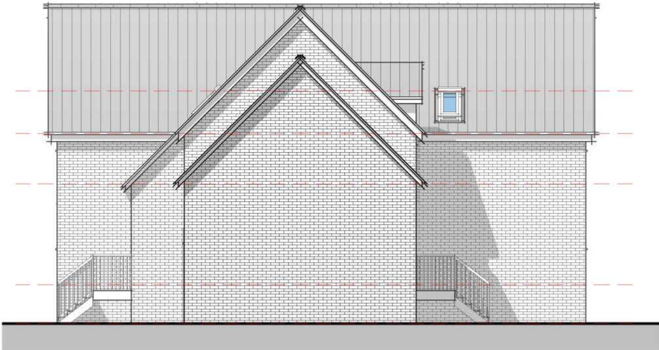
Elevation 02 - Right 1 : 100
