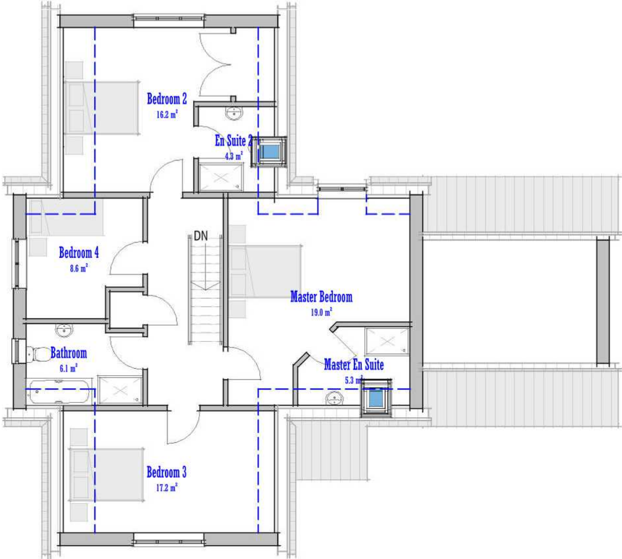
Plan 02 - First 1 : 100
