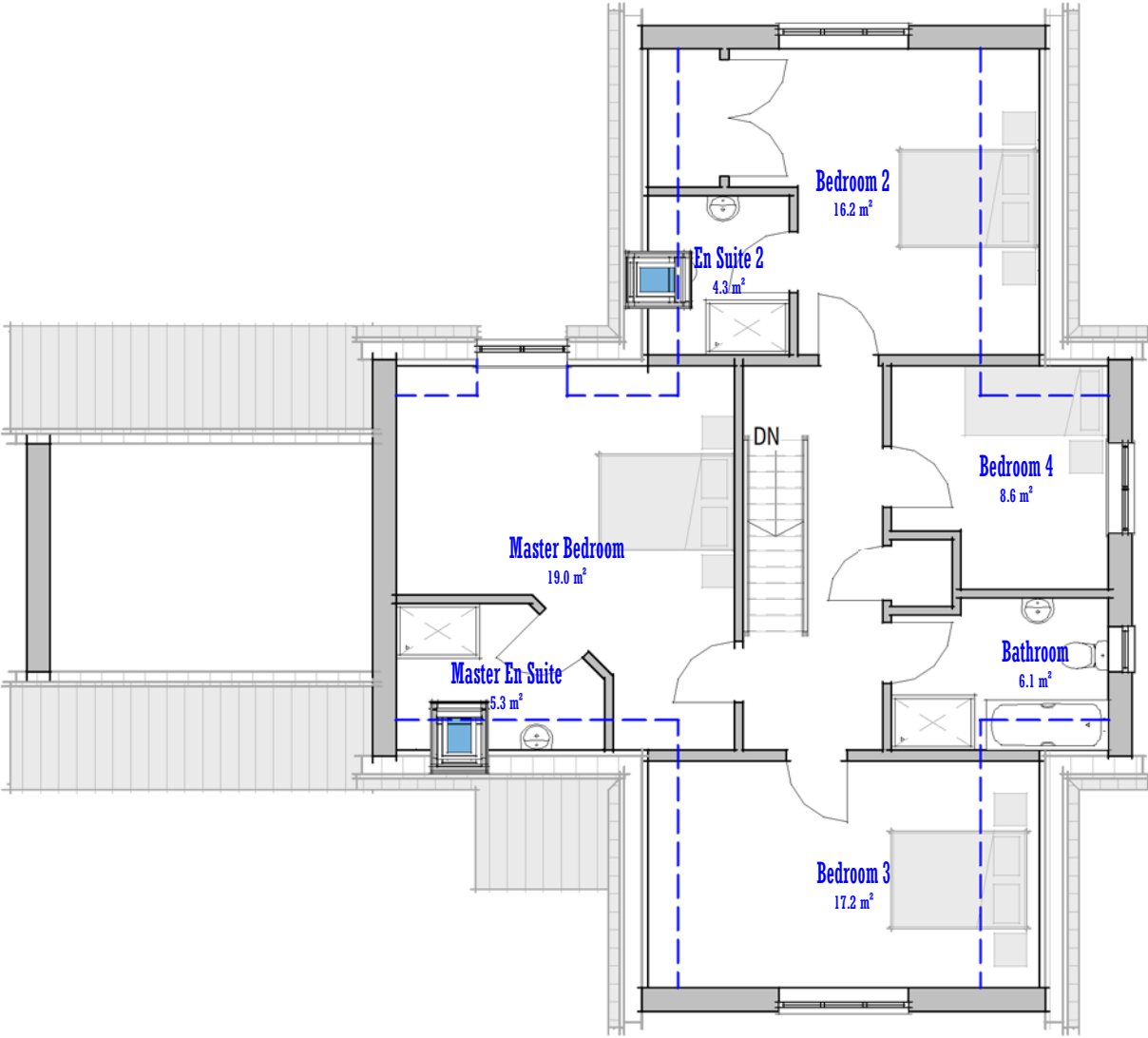
Plan 02 - First 1 : 100
