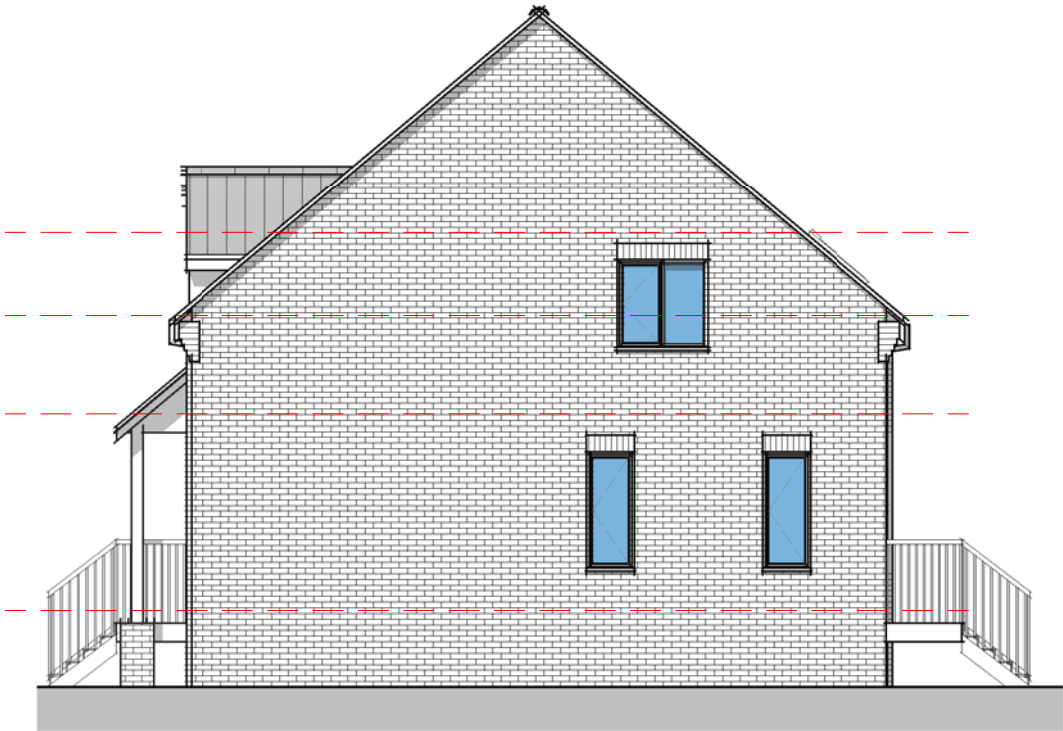
02 Elevation - Right
