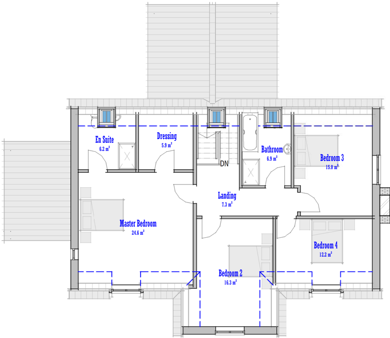
Plan 02 - First 1 : 100
