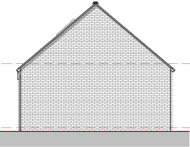
Elevation 05 - Left 1 : 100
