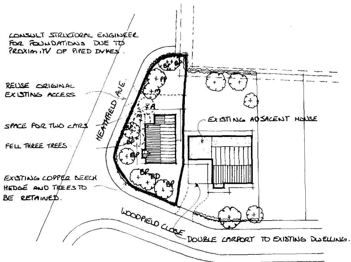
SITE PLAN 1:500
