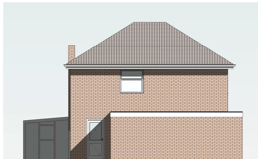
East 1 : 100
