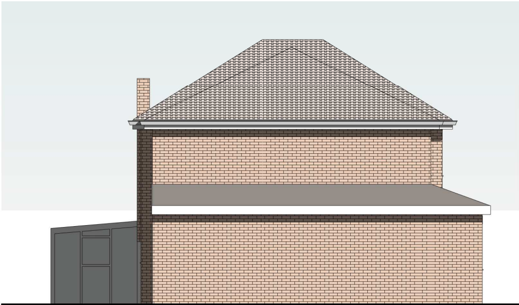
East 1 : 100
