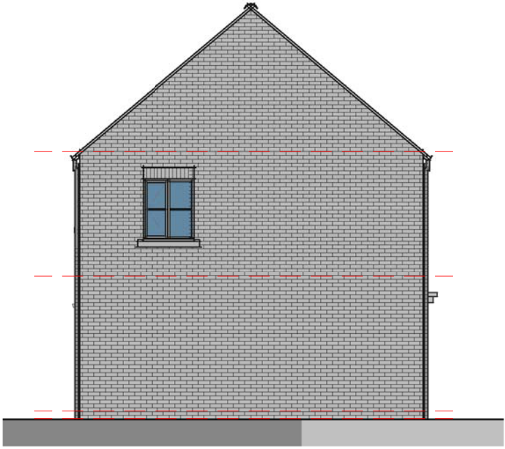
Elevation 04 - Left 1 : 100
