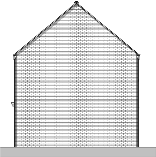
Elevation 02 - Right 1 : 100
