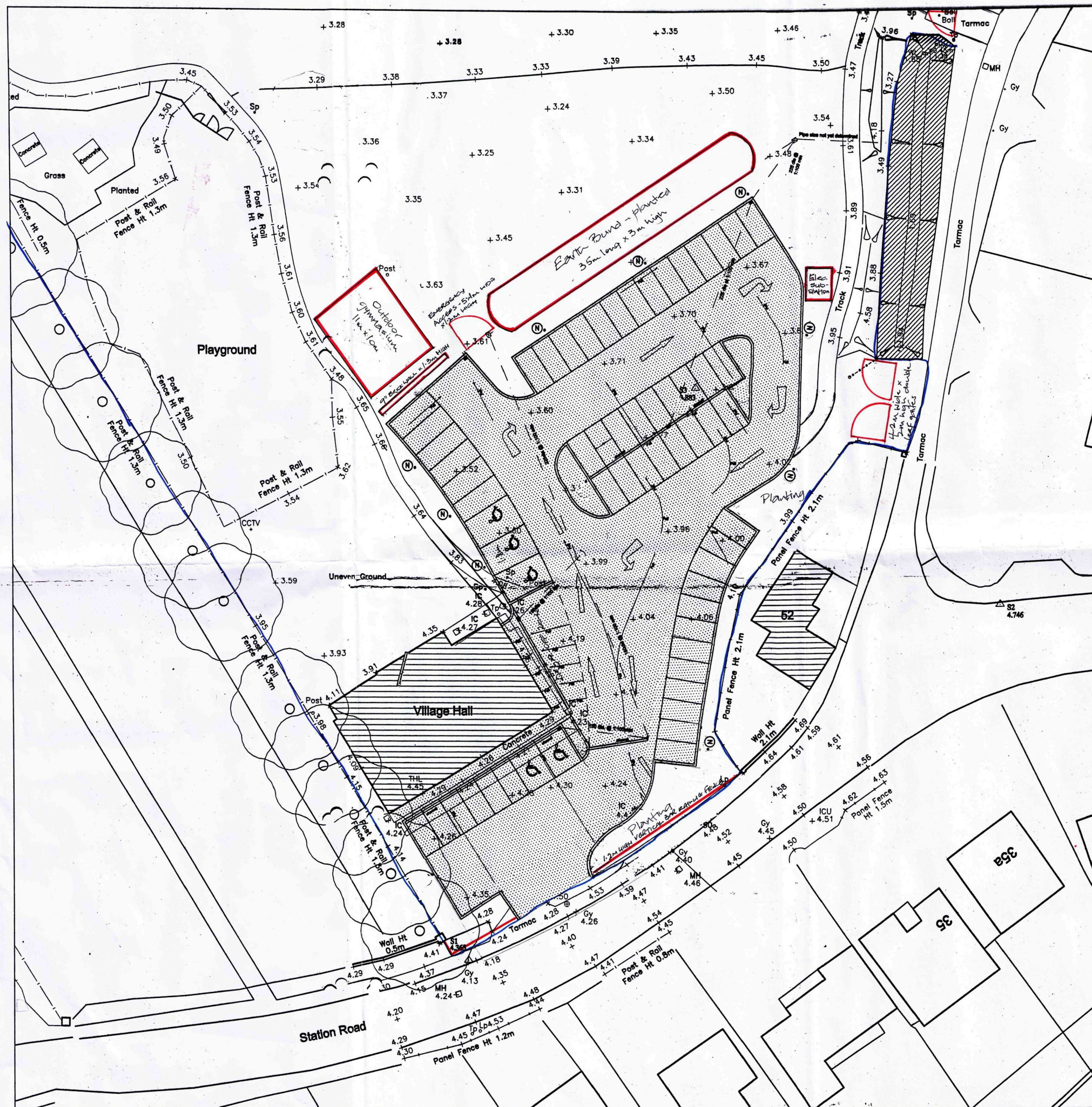
Site Layout Plan 1:250
