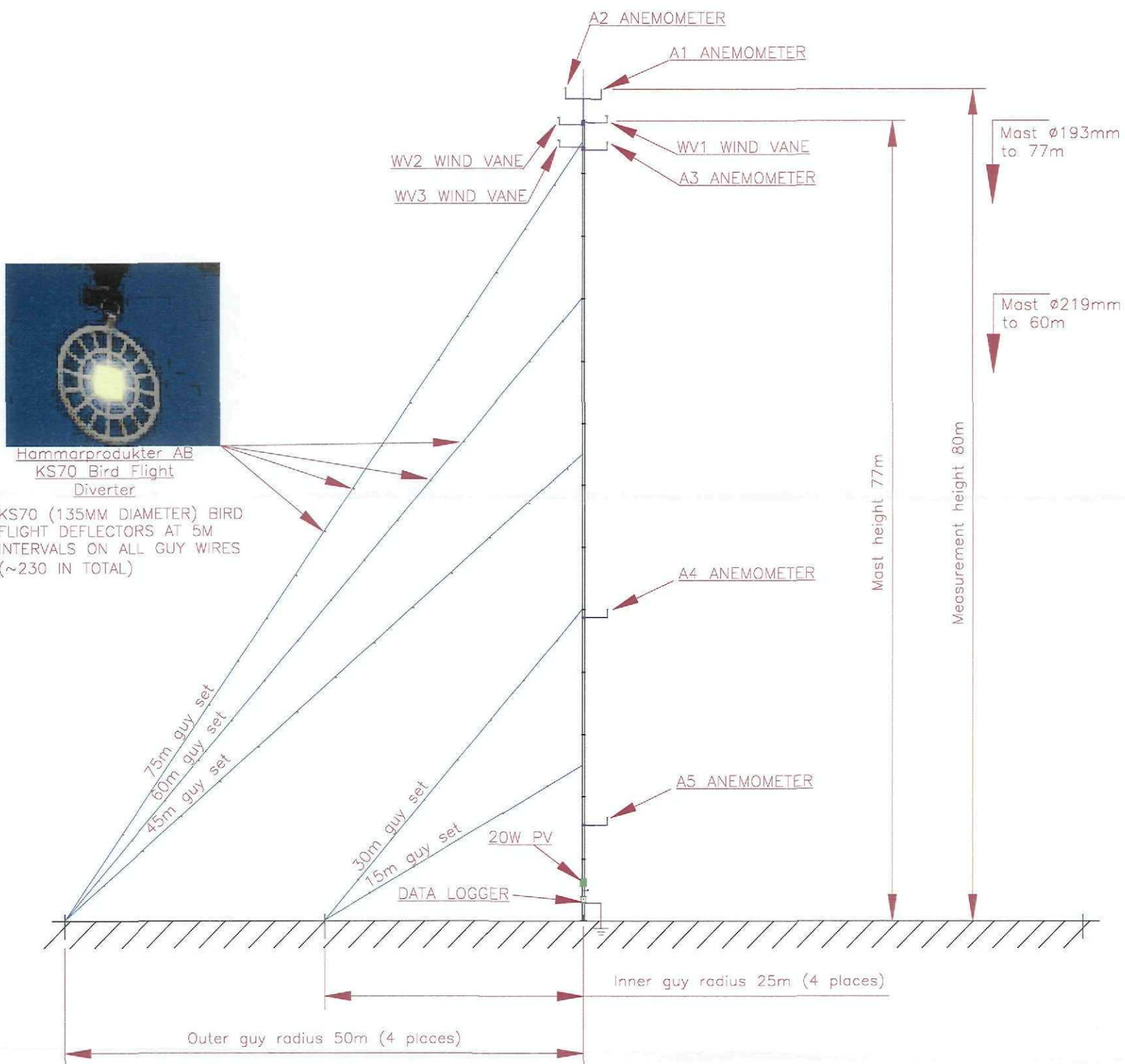
END ELEVATION
