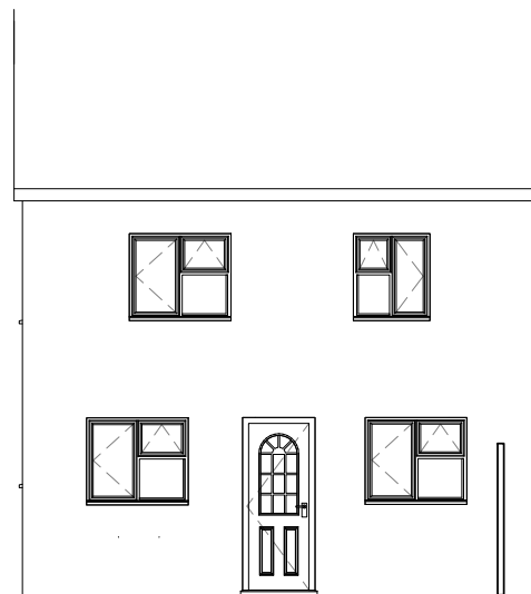
3 SE Elevation - (Existing) 1 : 100
